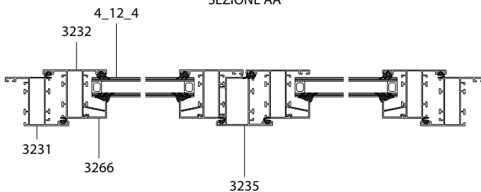
SEZIONE AA
