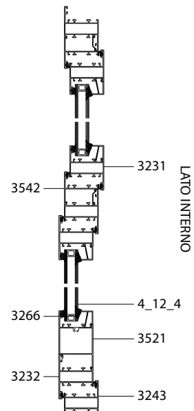
SEZIONE BB
